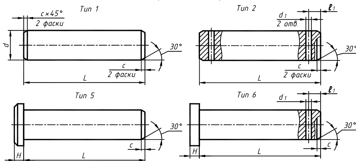
Оси (ГОСТ 9650-80)
